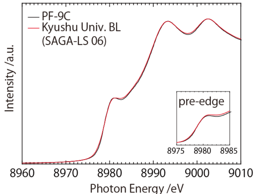
Cu foil Cu K-edge XANES spectra
