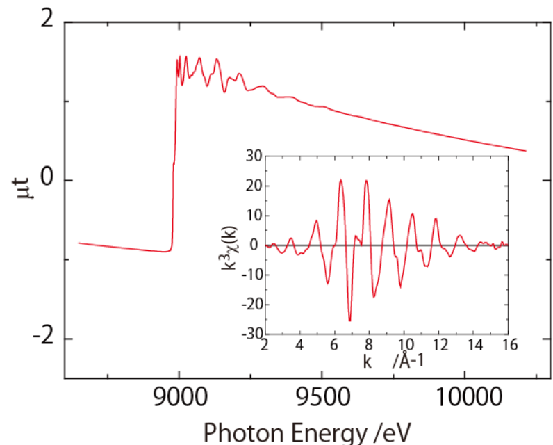
Cu foil Cu K-edge EXAFS spectrum
